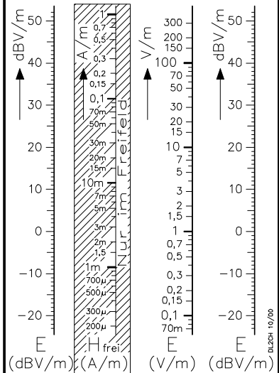
Umrechnungsskala für dBV => V
