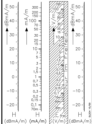
Umrechnungsskala für dBmA => mA
